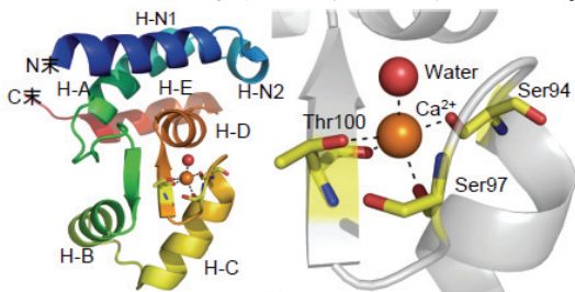
図3. Ca 2+ 結合型mIba1の全体構造(左)およびCa 2+ 結合部位の構造(右)。
